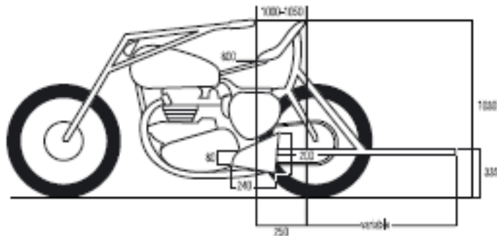
Dimensions en mm
